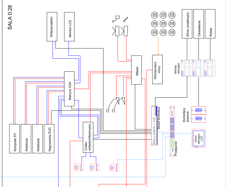
Schemat ideowy systemu AV
