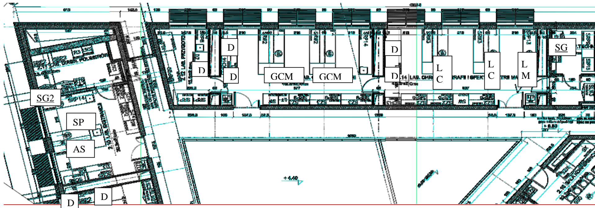
Schemat punktów doprowadzenia gazów technicznych wysokiej czystości (instalacja ze stali kwasoodpornej na zaciskach swagelok)
